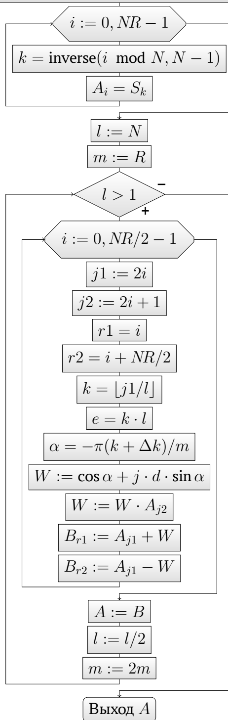
Рисунок А.1 – Алгоритм БПФ с прореживанием по времени, обратной перестановкой битов и дополнительным массивом. Авторский материал
