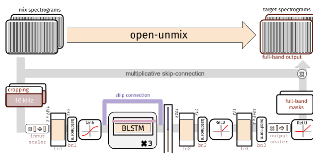
Рисунок 1.2 – Архитектура модели Open-Unmix [7]
