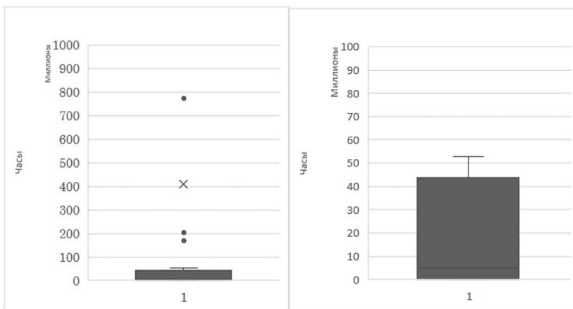
Рисунок 1. Распределение данных по переменной "Таймспент" (второй рисунок представлен без учета выбросов)
