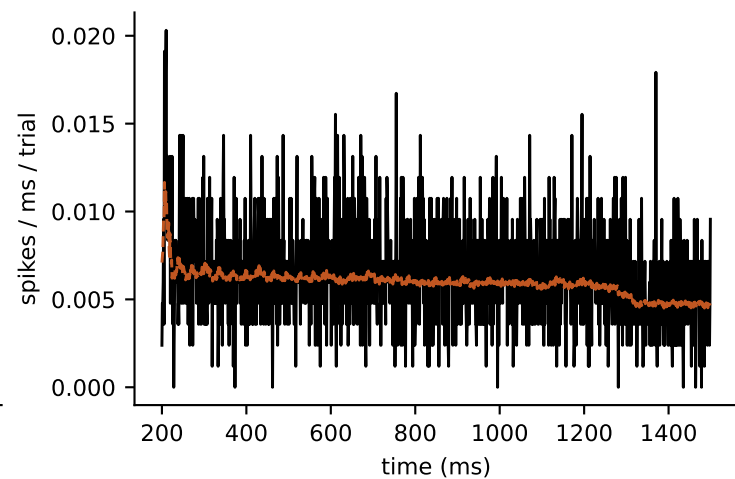
SOM mean PSTH (n=837)
