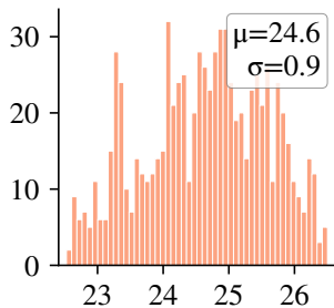
TMAX (°C)
