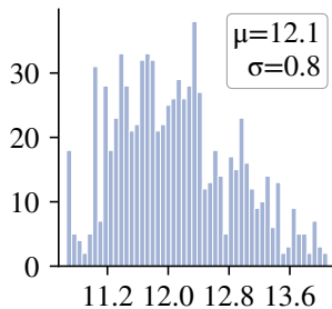
TMIN (°C)
