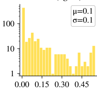
SWE (kg/m 2 )
