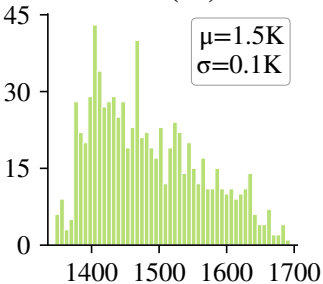
VP (Pa)
