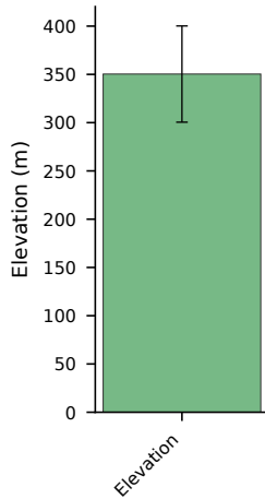
DEM
