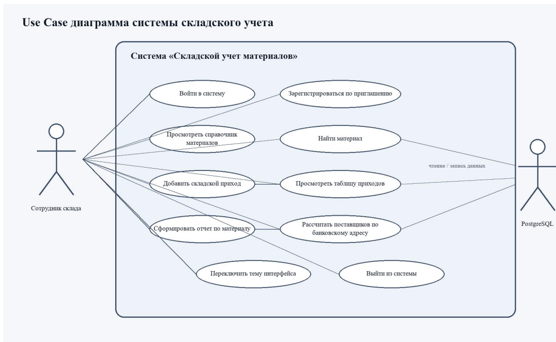
Рисунок 2.1 - Use Case диаграмма системы складского учета материалов
