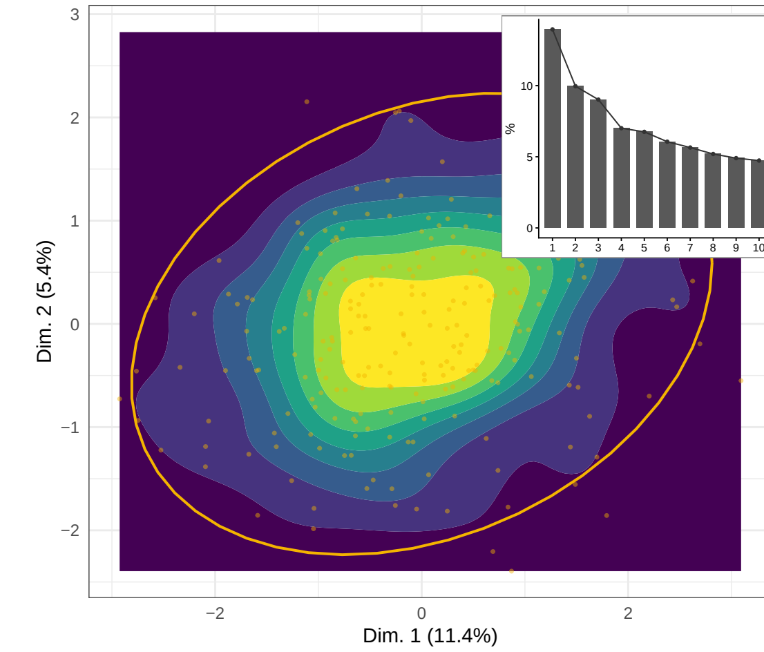
B celltype_2 · Thomson FA
