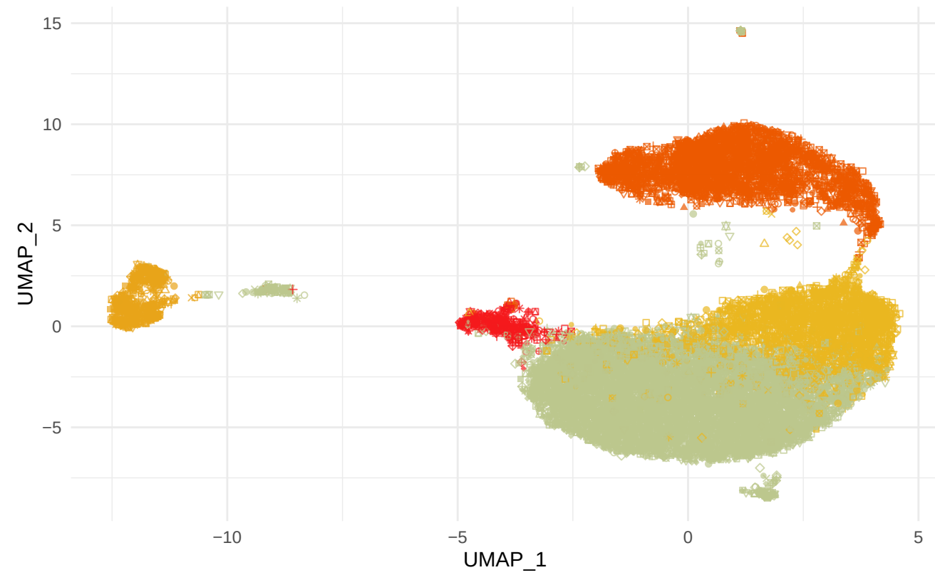
UMAP
