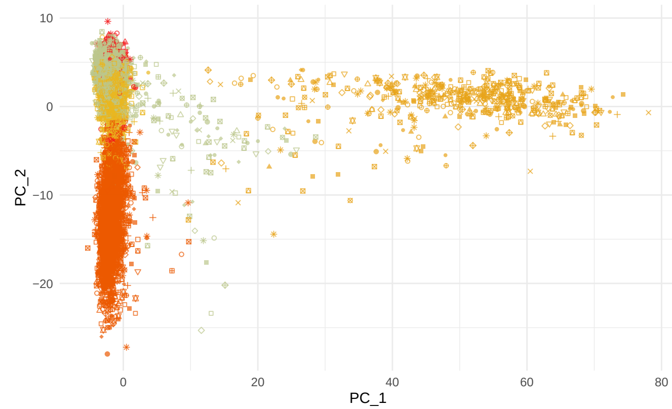
PCA
