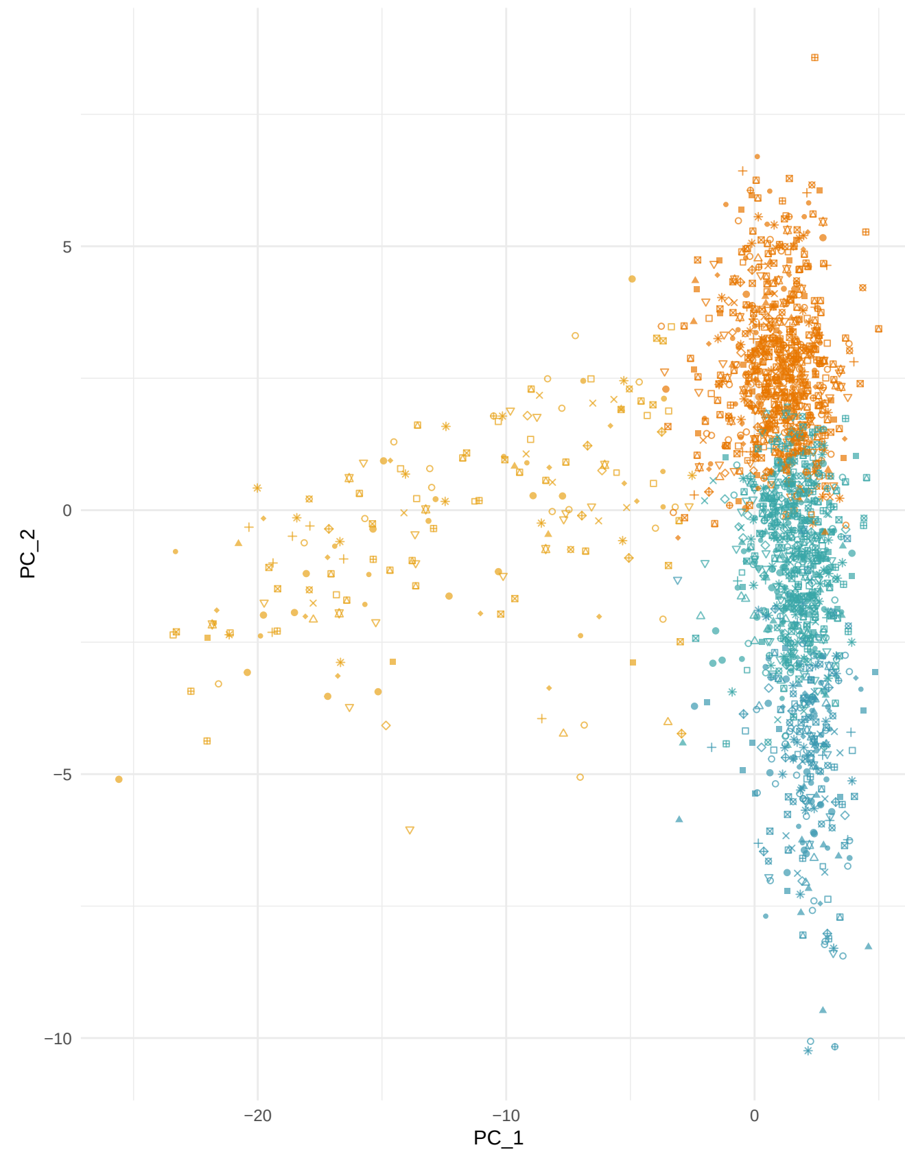
PCA
