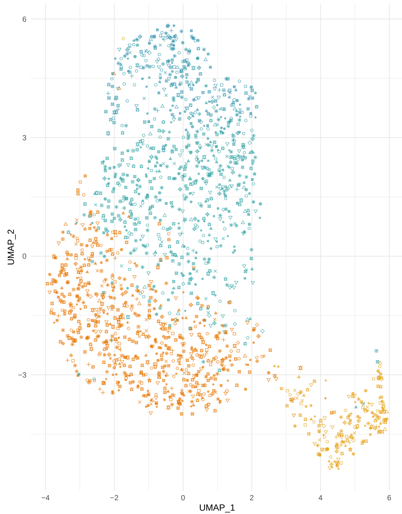
UMAP
