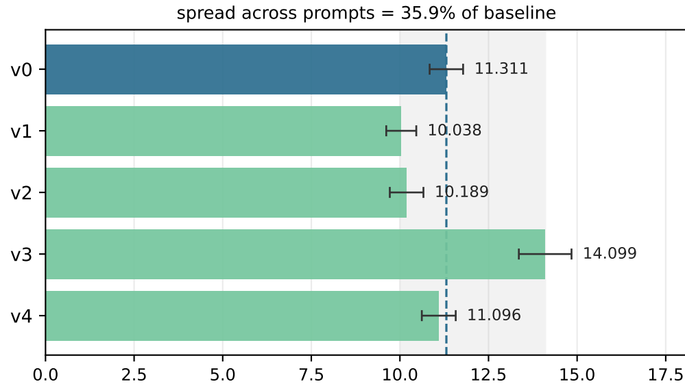
GPT-4.1 Mini
