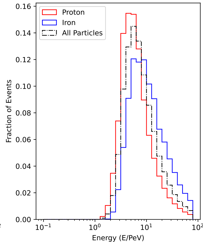
6.6 PeV
