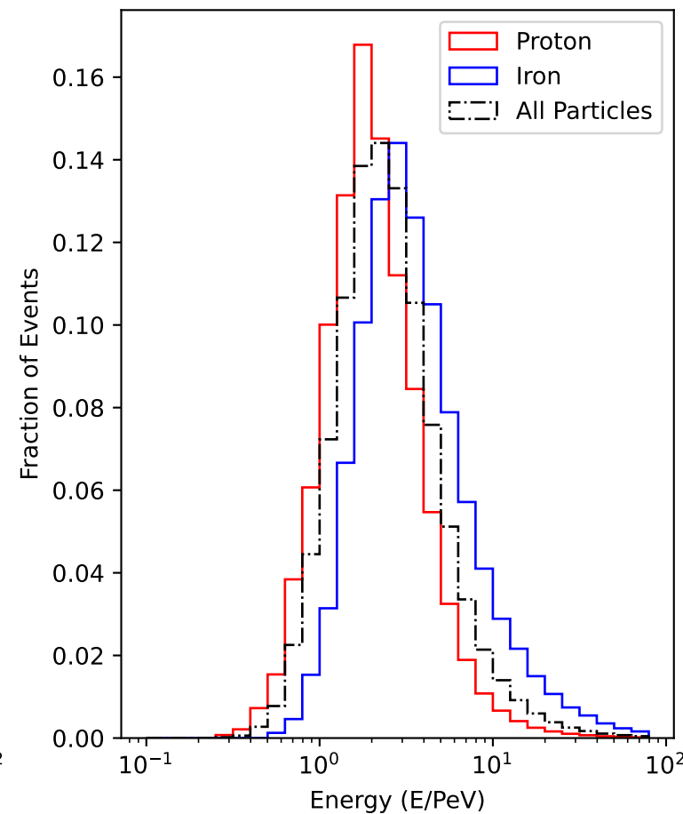
2.3 PeV
