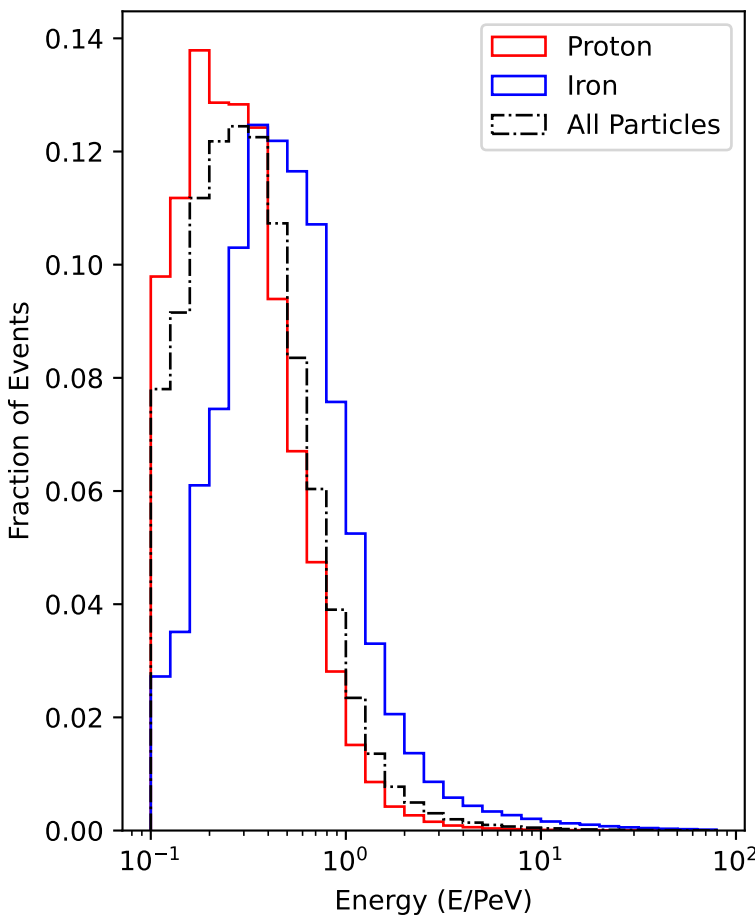
300 TeV
