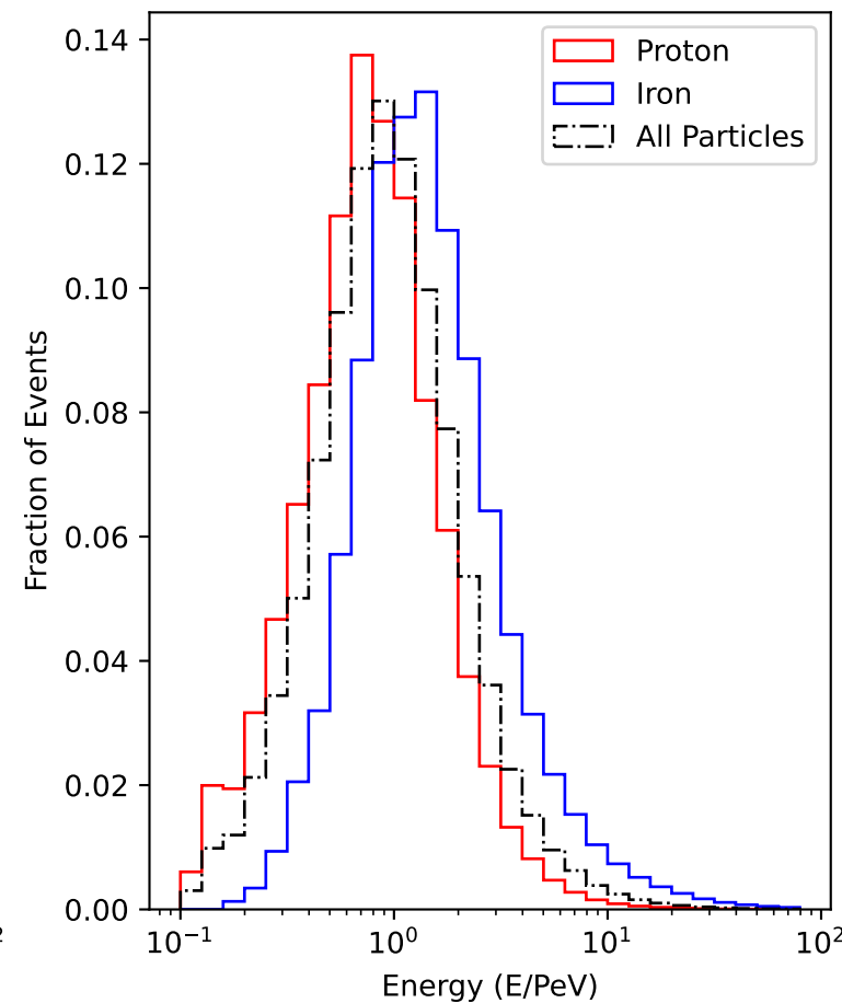
900 TeV
