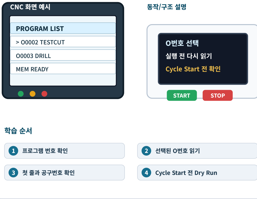
그림 8-2. 프로그램 호출의 CNC 화면 예시, 조작 순서, 실제 움직임을 함께 보는 학습용 도해.
