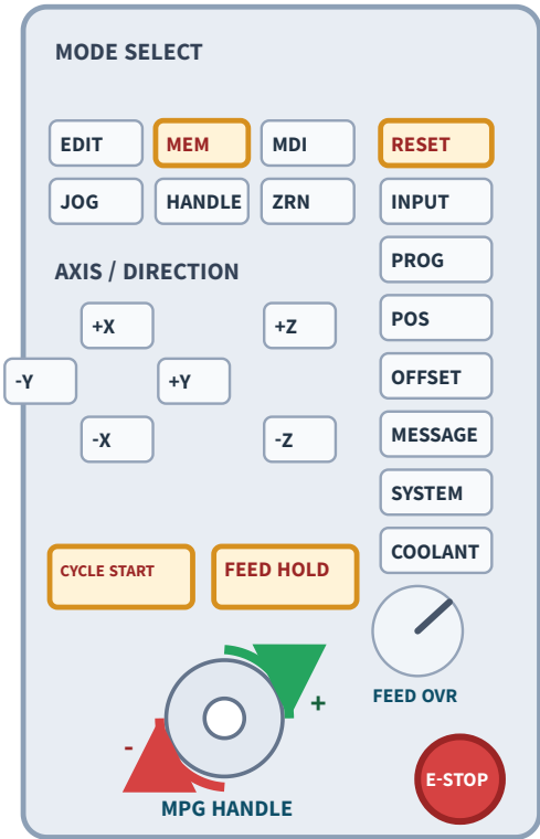
Hình 20-2. Mockup màn hình CNC và bảng điều khiển cần đọc trong bài Thực hành gia công đầu tiên.
