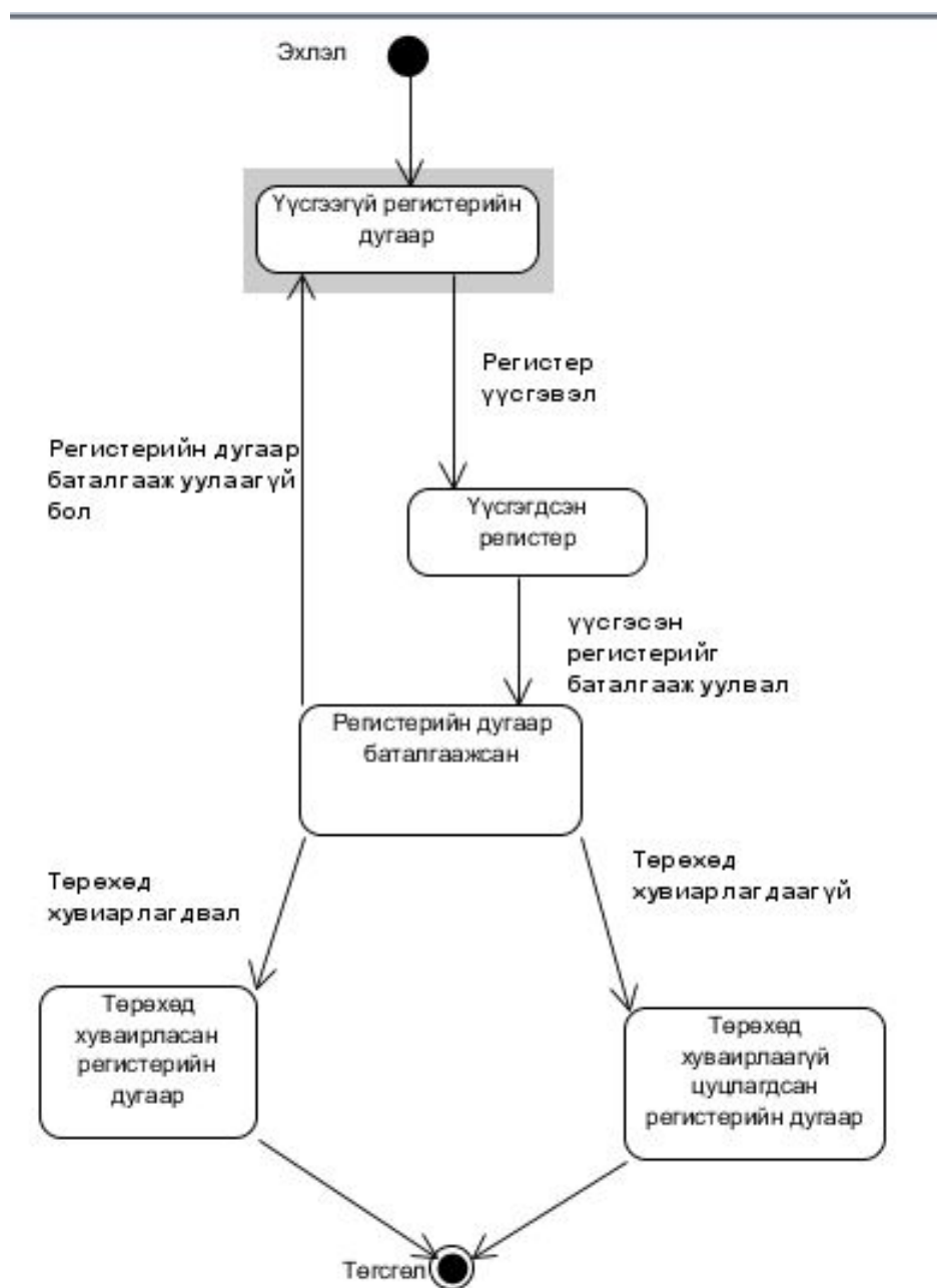
ЗУРАГ 3.11: Регистрийн дугаар үүсгэх төлөв шилжилтийн диаграм
