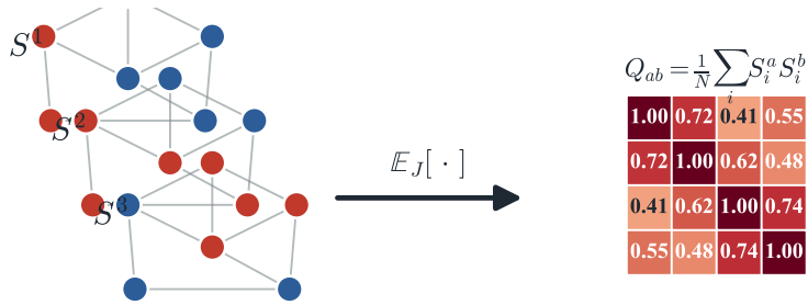
(d) Replica method: n copies share one J
