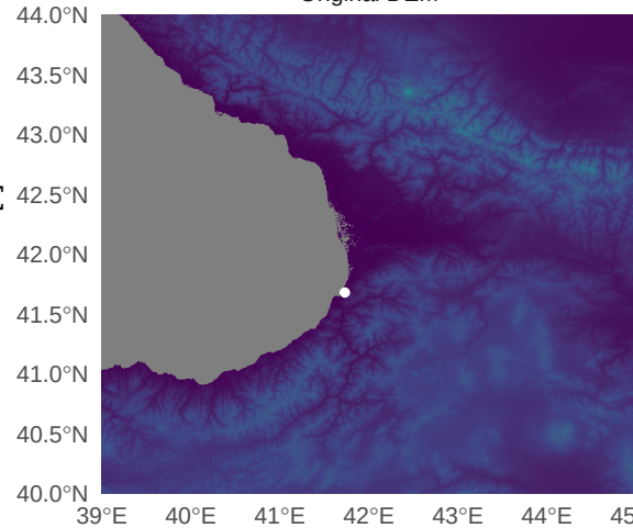
Original DEM
