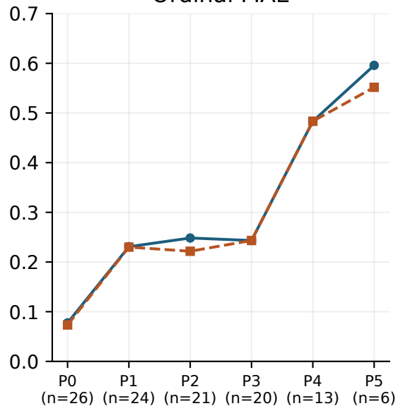
Ordinal MAE
