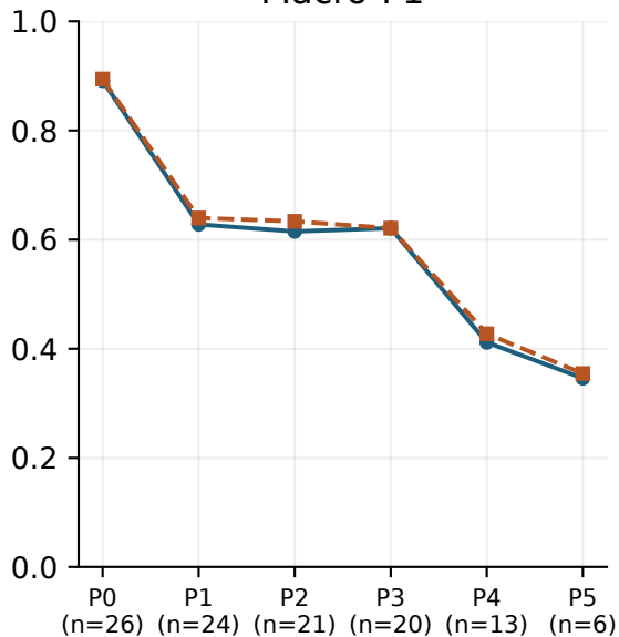
Macro-F1
