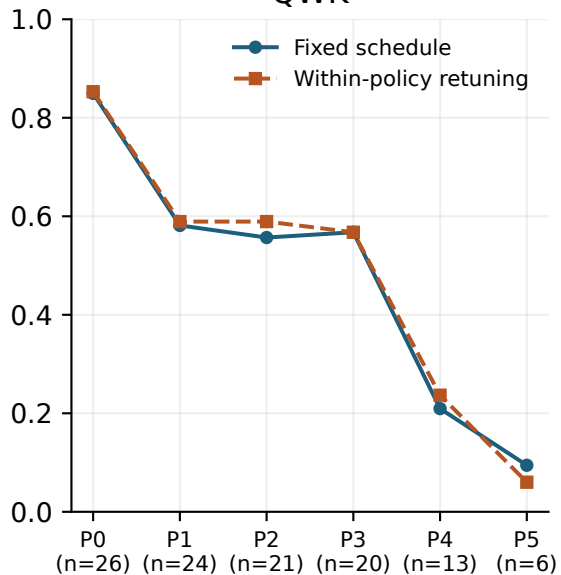
QWK
