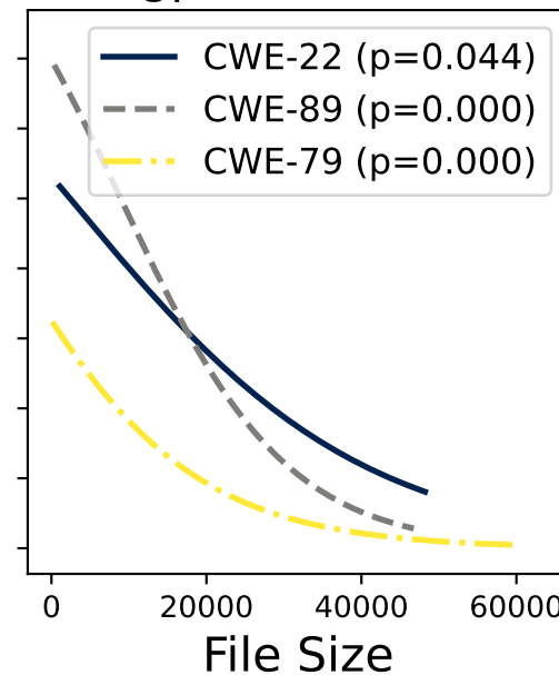
gpt-3.5-turbo
