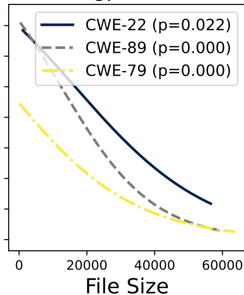
gpt-4o
