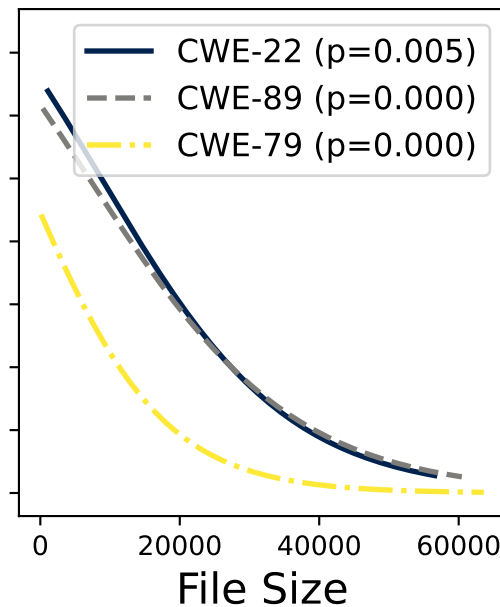
mixtral-8x22b
