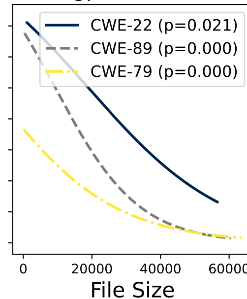
gpt-4-turbo
