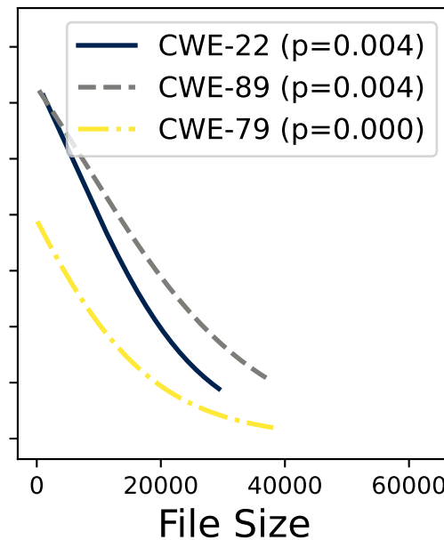
llama-3-70b
