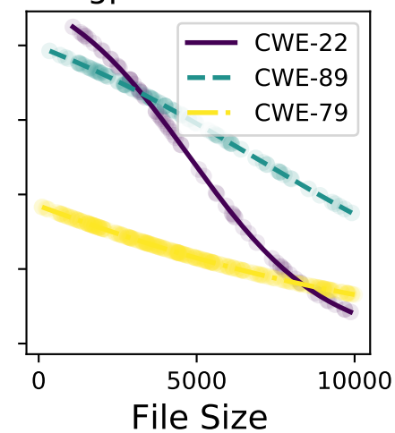
gpt-3.5-turbo
