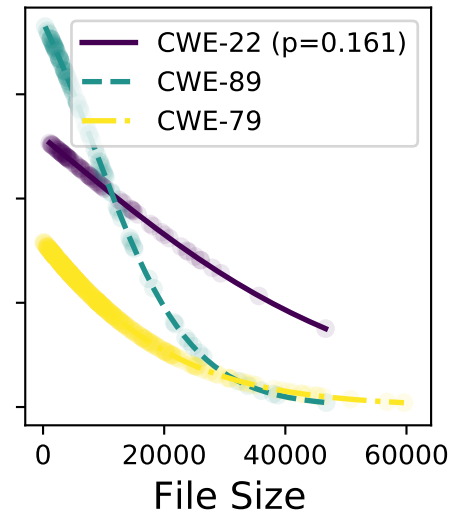
gpt-3.5-turbo
