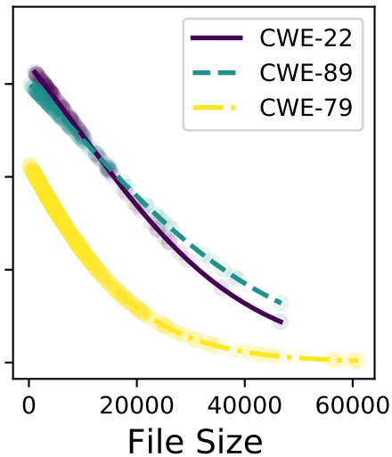
mixtral-8x22b
