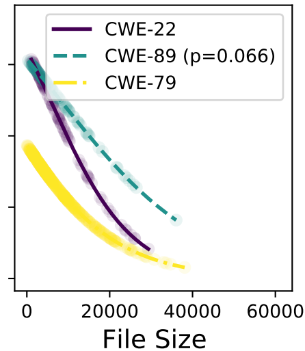
llama-3-70b
