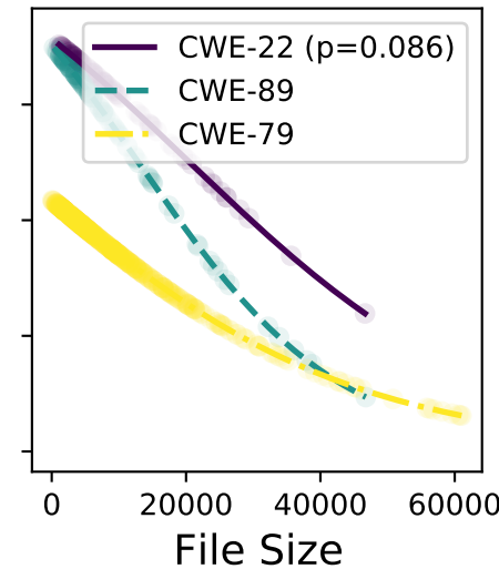
gpt-4o
