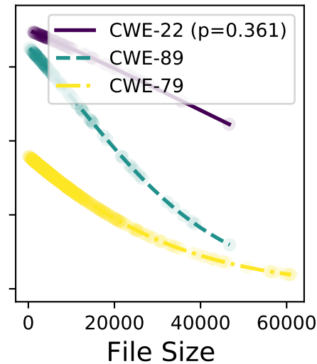
gpt-4-turbo
