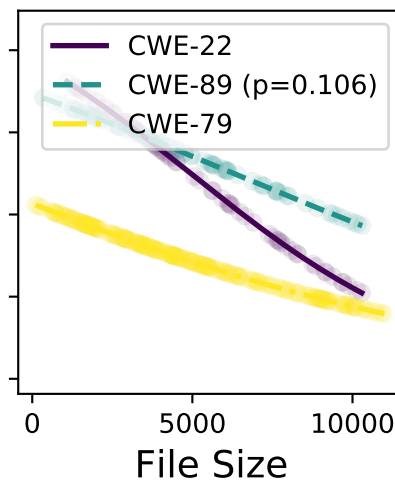
llama-3-70b
