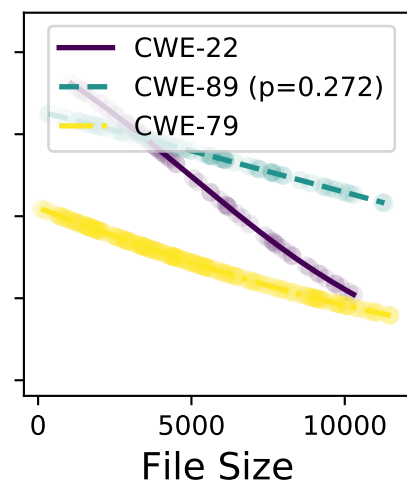
llama-3-70b
