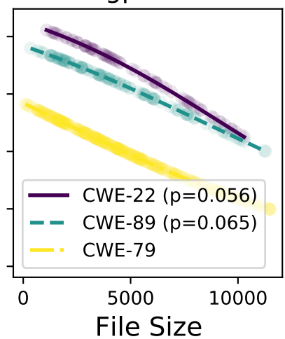
gpt-4o
