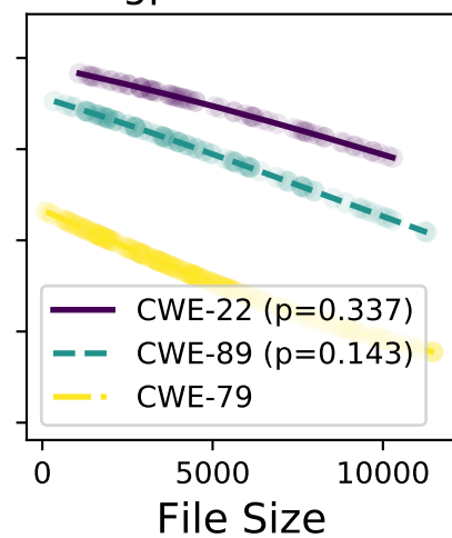
gpt-4-turbo
