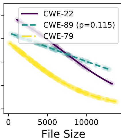
mixtral-8x22b
