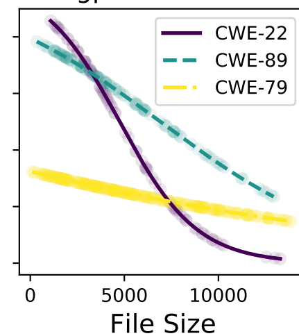
gpt-3.5-turbo
