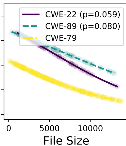
llama-3-70b
