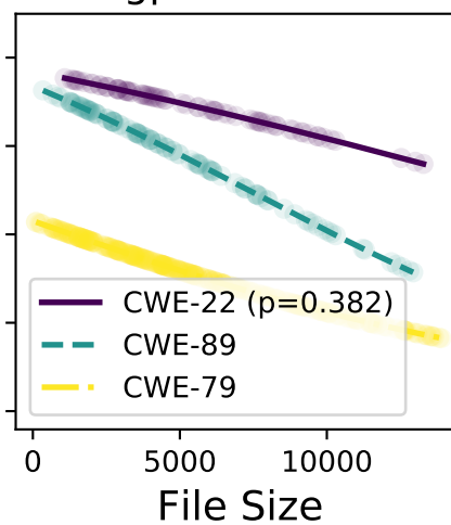
gpt-4-turbo
