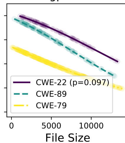
gpt-4o
