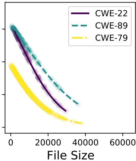
llama-3-70b
