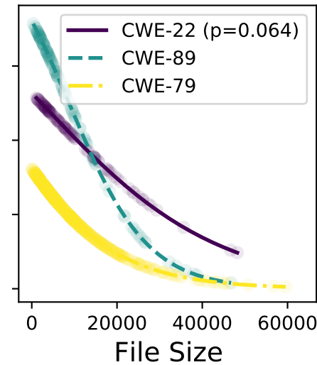
gpt-3.5-turbo
