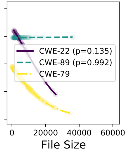
llama-3-70b
