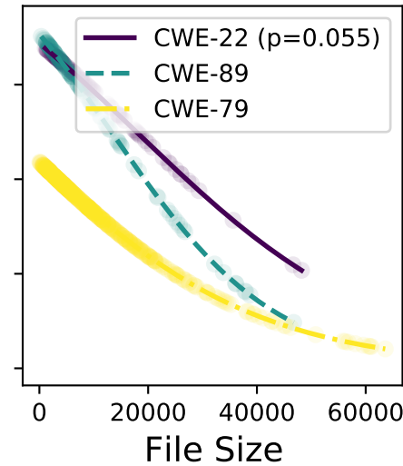
gpt-4o
