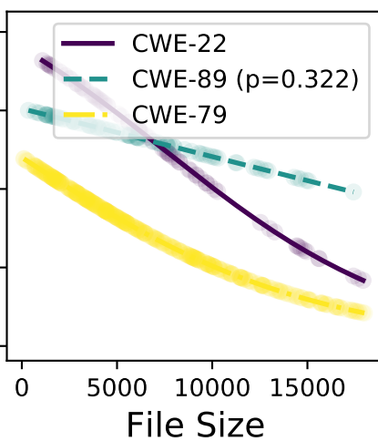
mixtral-8x22b
