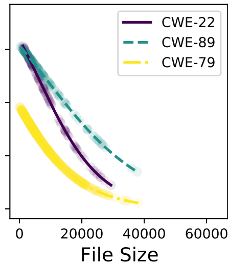
llama-3-70b
