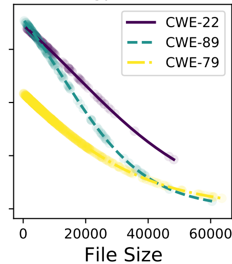
gpt-4o
