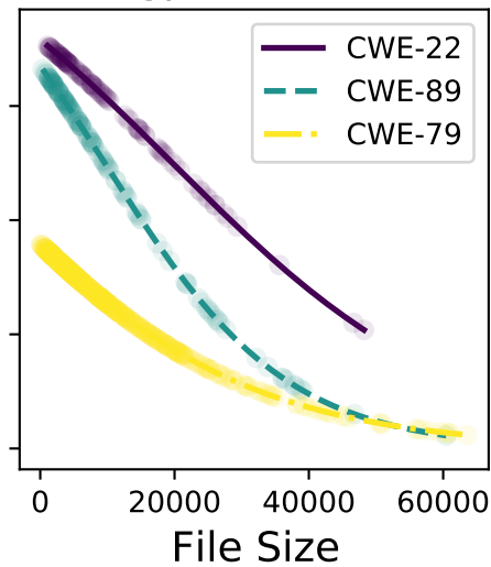
gpt-4-turbo
