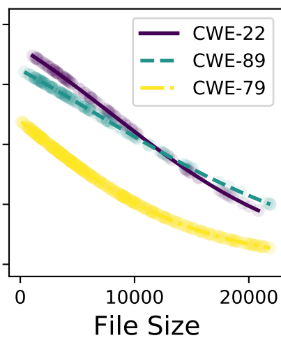
mixtral-8x22b
