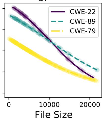
gpt-4o
