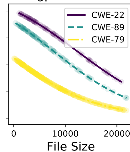
gpt-4-turbo
