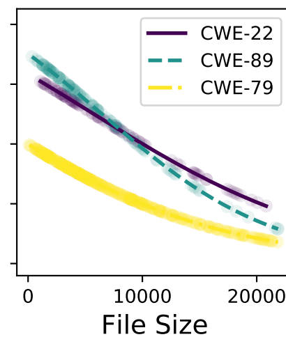
llama-3-70b
