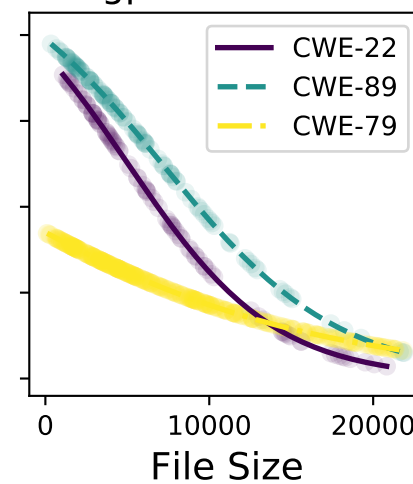
gpt-3.5-turbo
