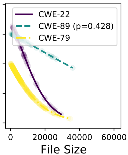
llama-3-70b
