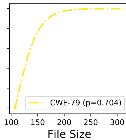
mixtral-8x22b
