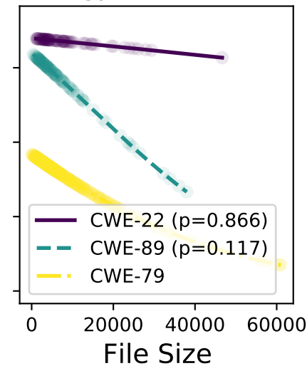
gpt-4-turbo
