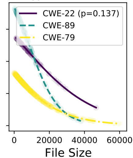
gpt-3.5-turbo
