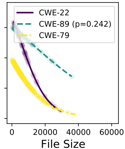
llama-3-70b
