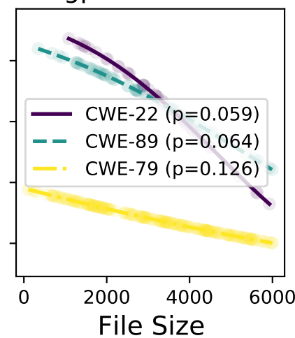
gpt-3.5-turbo
