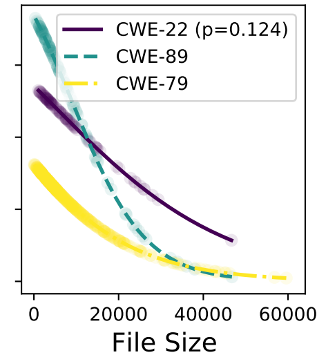
gpt-3.5-turbo
