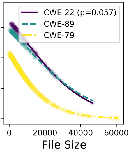
mixtral-8x22b
