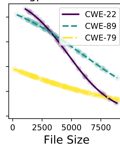
gpt-3.5-turbo
