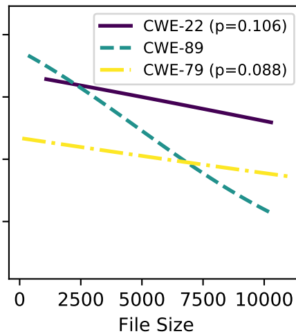
llama-3-70b
