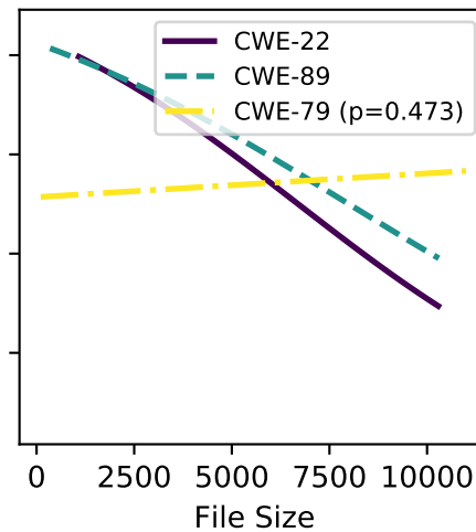
gpt-4-turbo
