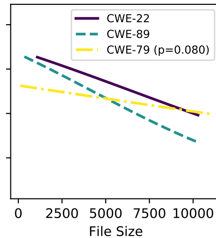
mixtral-8x22b
