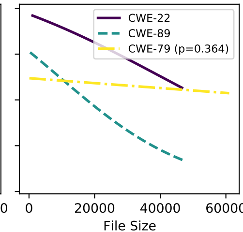
gpt-4o
