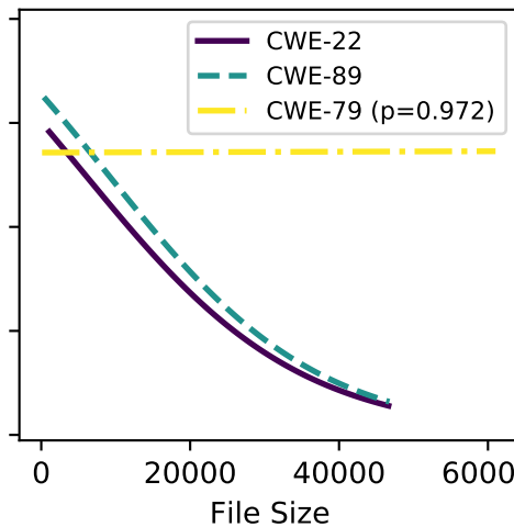
gpt-4-turbo
