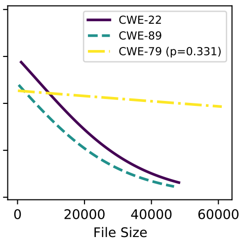
mixtral-8x22b
