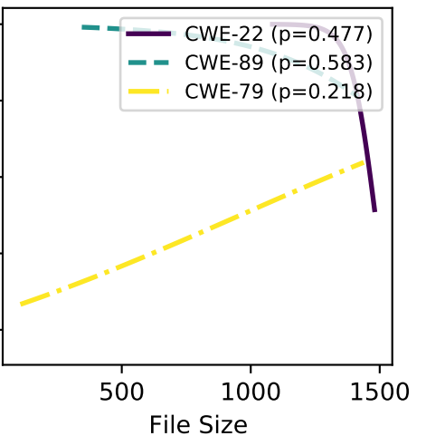
gpt-4o
