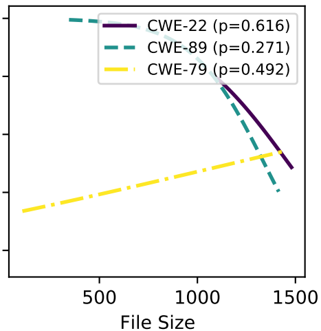
llama-3-70b
