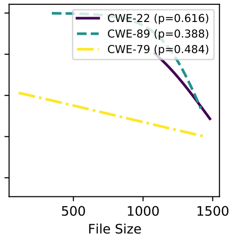
mixtral-8x22b
