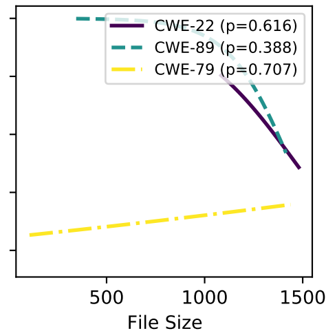
gpt-3.5-turbo
