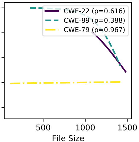
gpt-4-turbo
