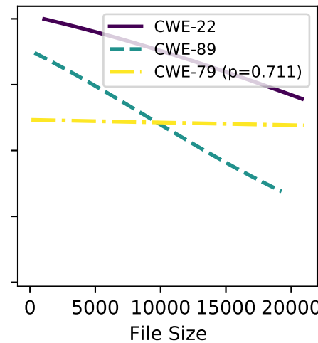
gpt-4o
