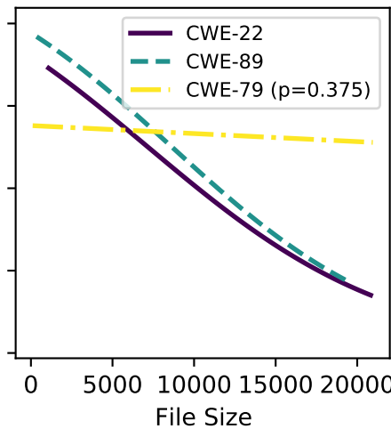
gpt-4-turbo
