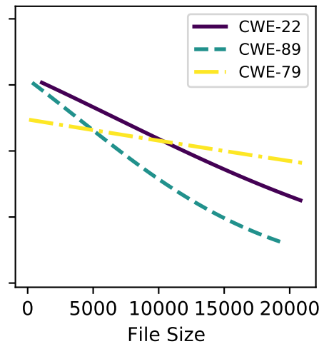
mixtral-8x22b
