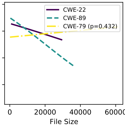
gpt-4-turbo
