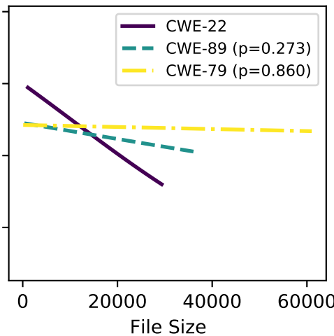
mixtral-8x22b
