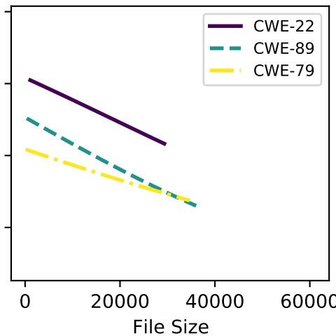
llama-3-70b
