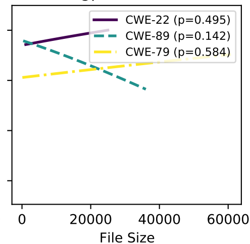
gpt-4-turbo
