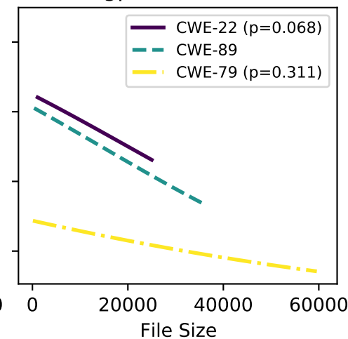
gpt-3.5-turbo
