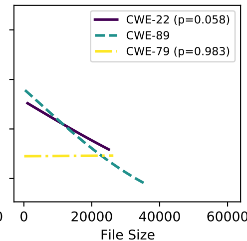
llama-3-70b
