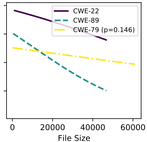
gpt-4o
