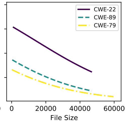
gpt-3.5-turbo
