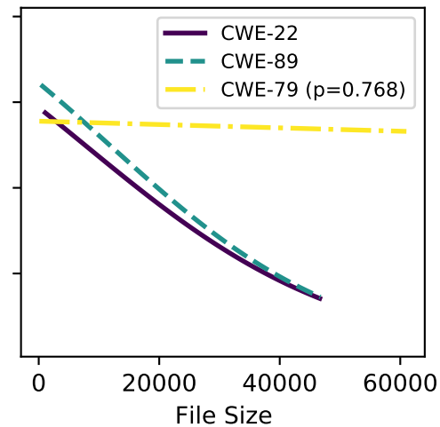
gpt-4-turbo
