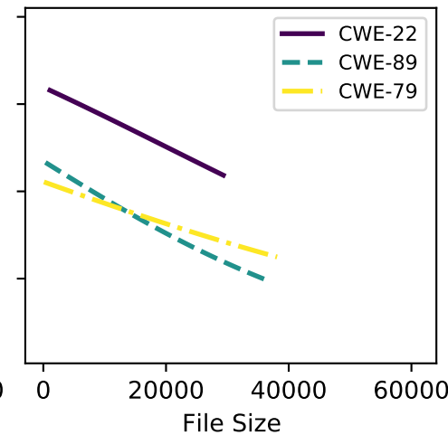
llama-3-70b
