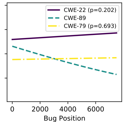
mixtral-8x22b
