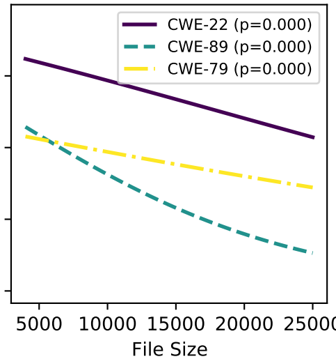
llama3-70b
