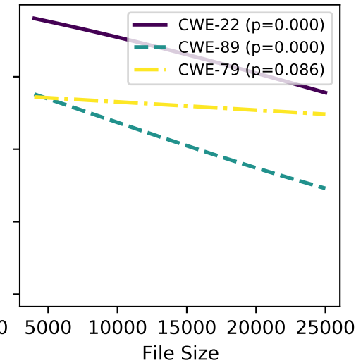
gpt-4o
