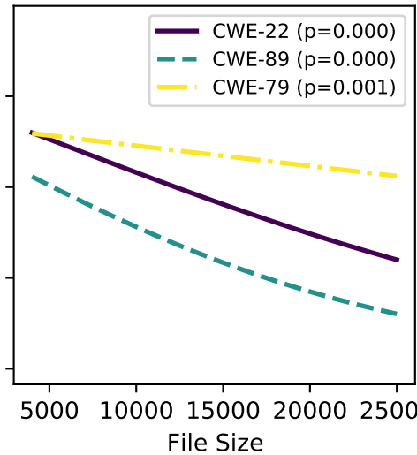
mixtral-8x22b
