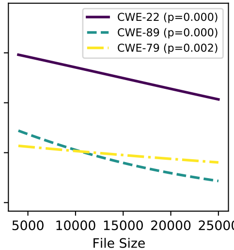
gpt-3.5-turbo
