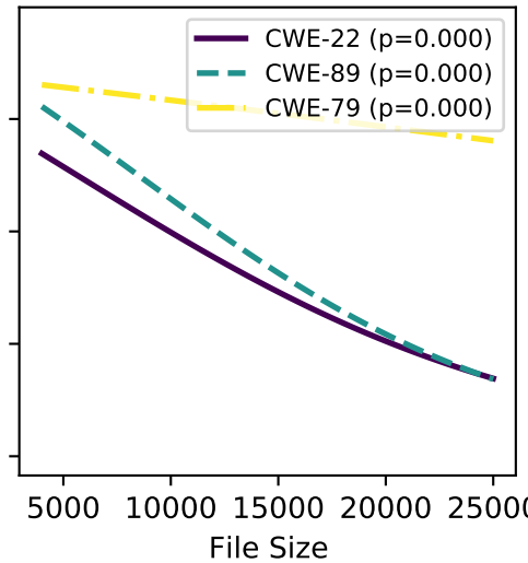
gpt-4-turbo
