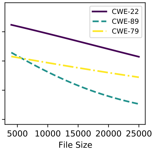
llama-3-70b
