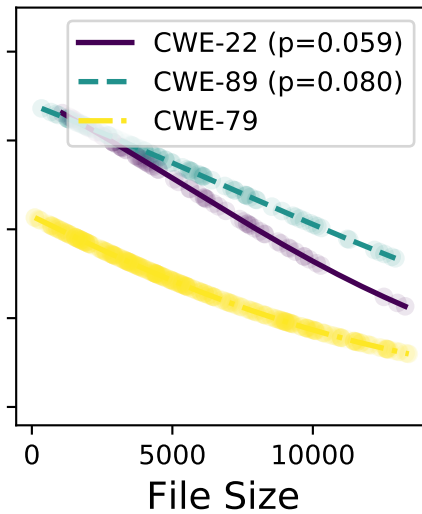
llama-3-70b-8192
