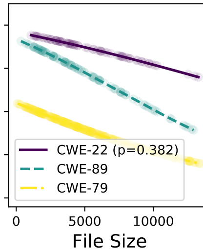
gpt-4-turbo
