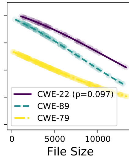
gpt-4o
