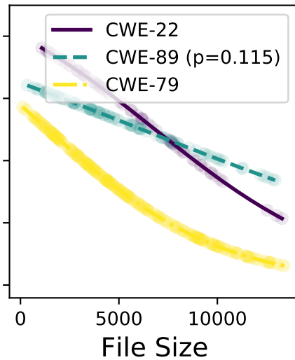
mixtral-8x22b
