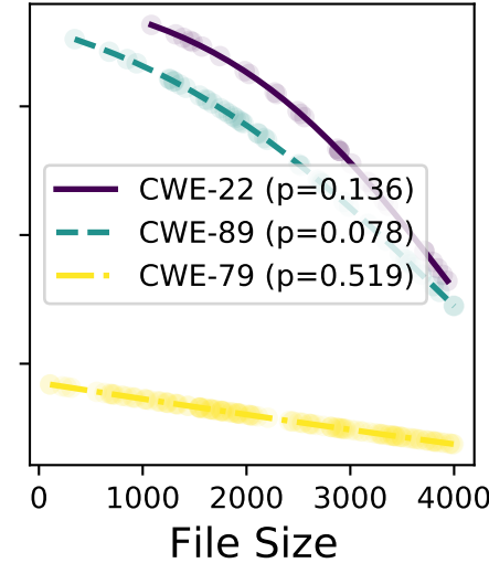
gpt-3.5-turbo
