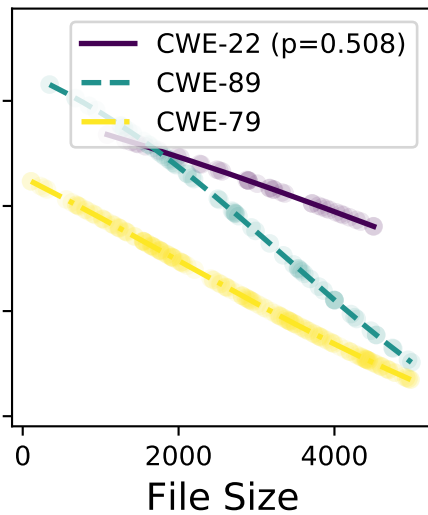
mixtral-8x22b
