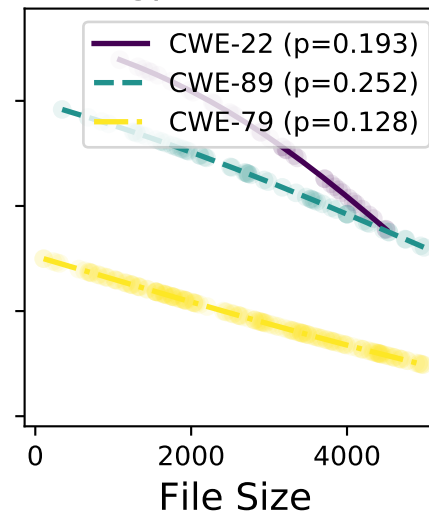
gpt-4-turbo
