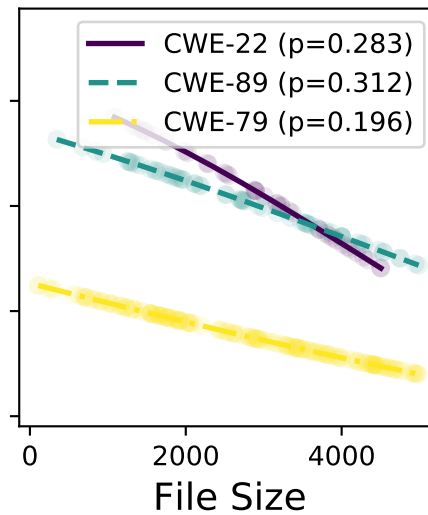
llama-3-70b-8192
