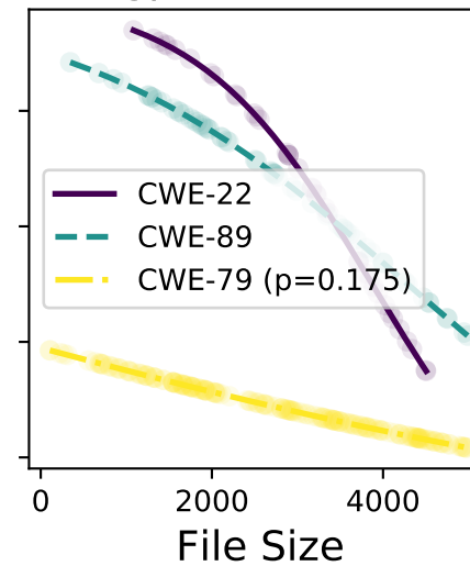
gpt-3.5-turbo
