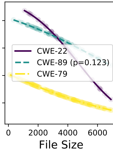
gpt-3.5-turbo
