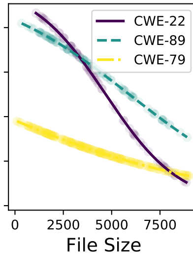
gpt-3.5-turbo
