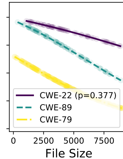
gpt-4-turbo
